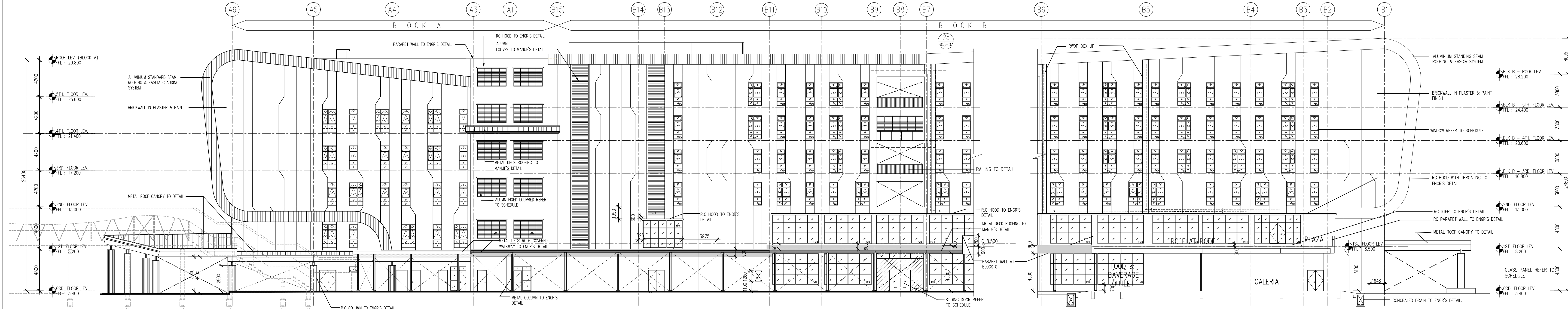
1a PANDANGAN UTARA - SKALA = 1 : 200
