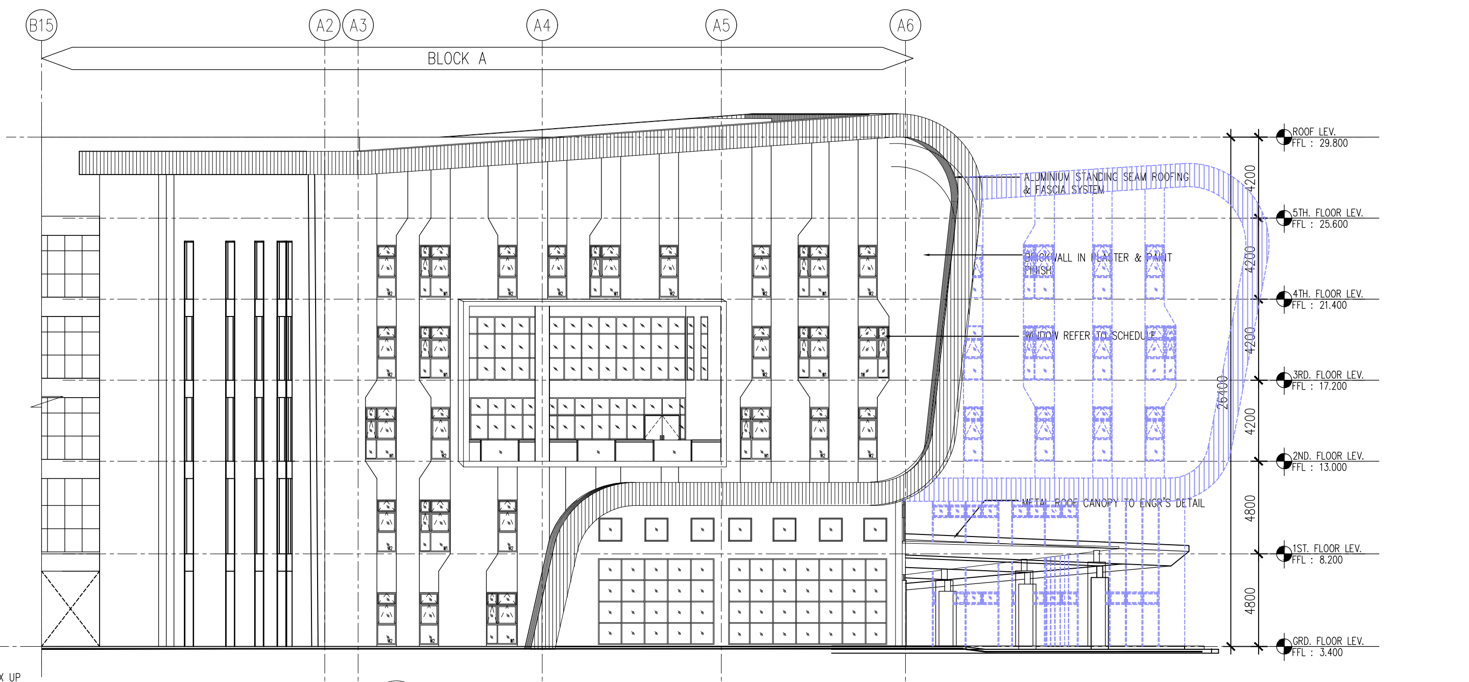
2b PANDANGAN SELATAN - SKALA = 1 : 200
