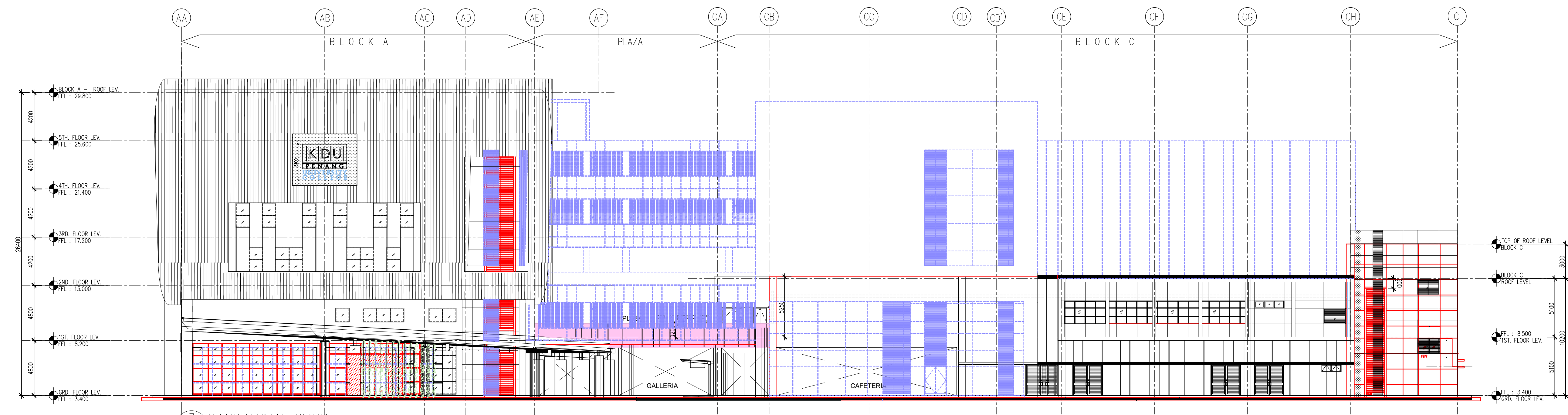
3 PANDANGAN TIMUR - SKALA = 1 : 200
