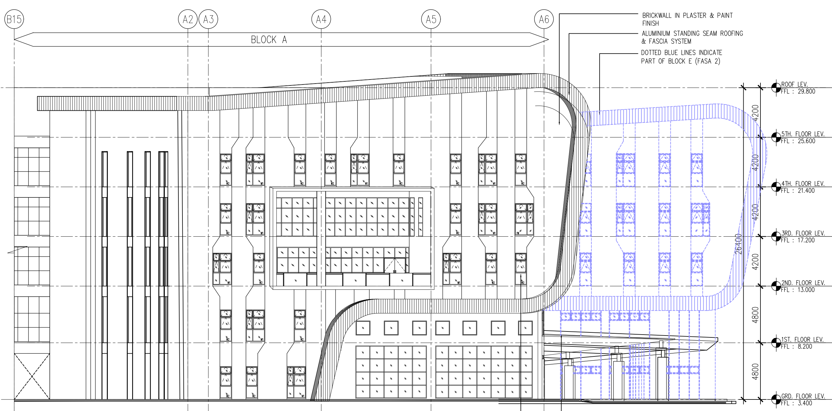
2b PANDANGAN SELATAN 201 SKALA = 1 : 200
