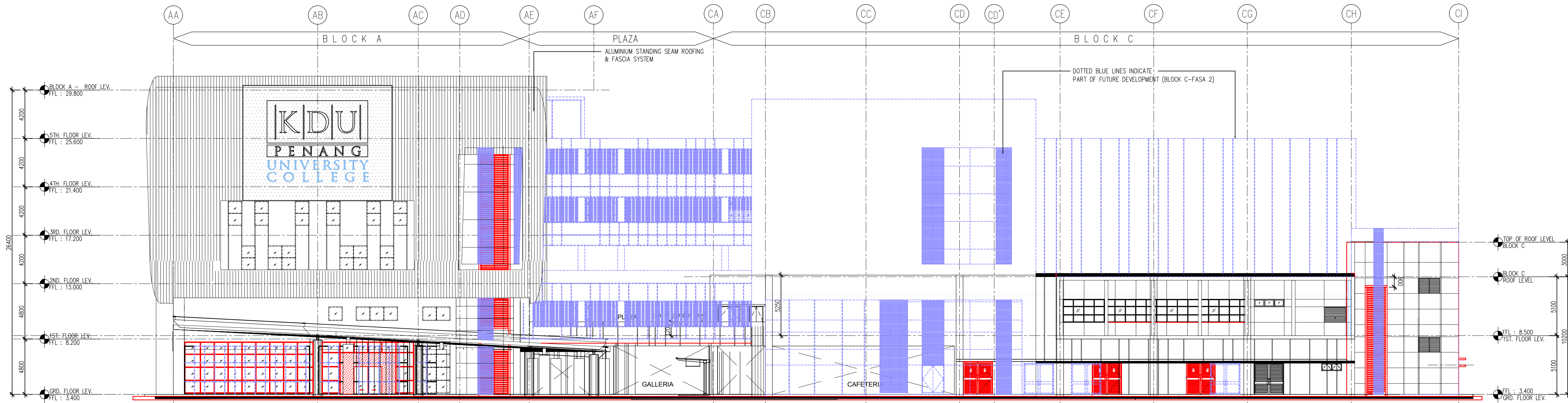
3 PANDANGAN TIMUR 201 SKALA = 1 : 200
