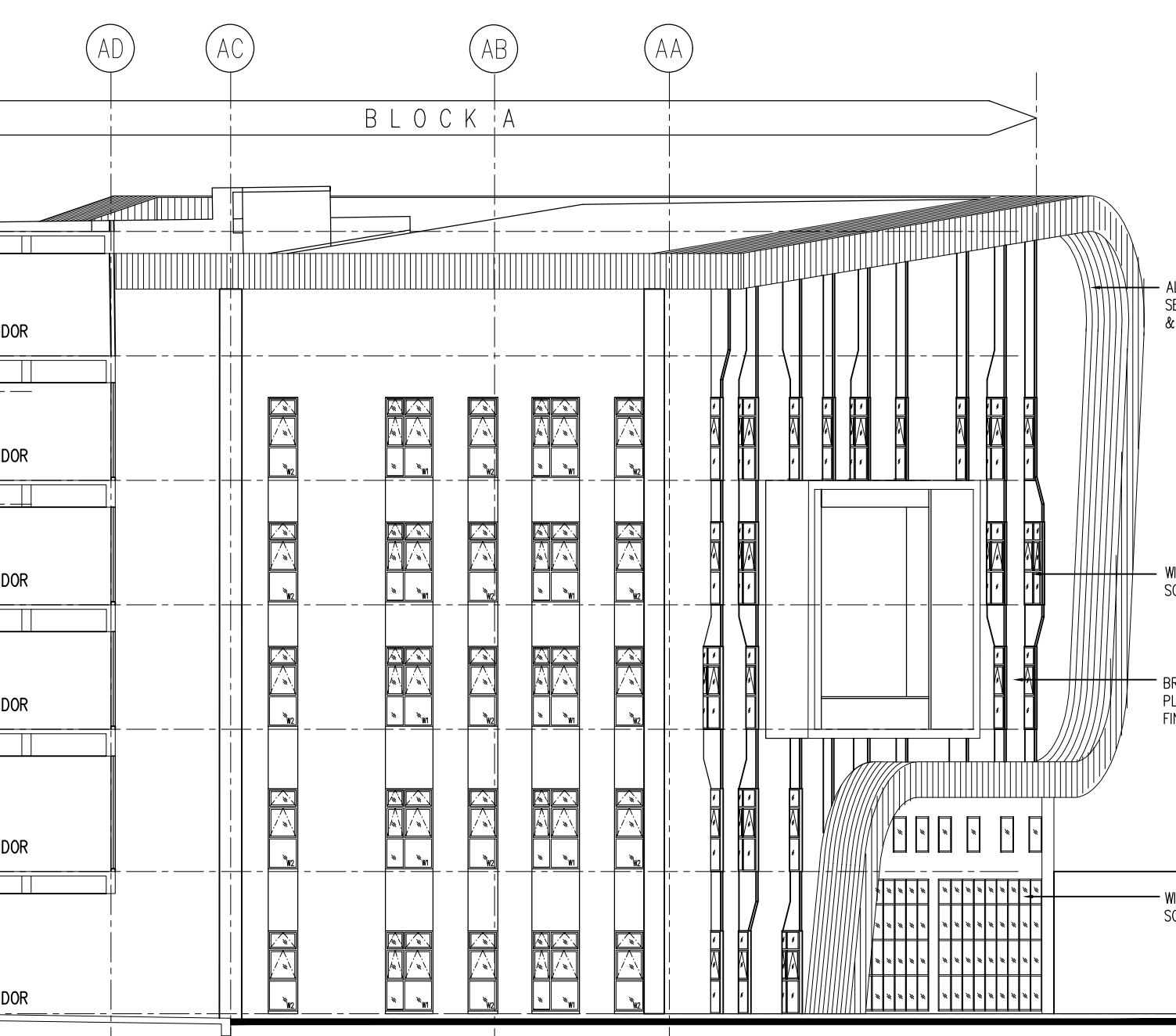
2c BLK. A - PANDANGAN BARAT 201 SKALA = 1 : 200
