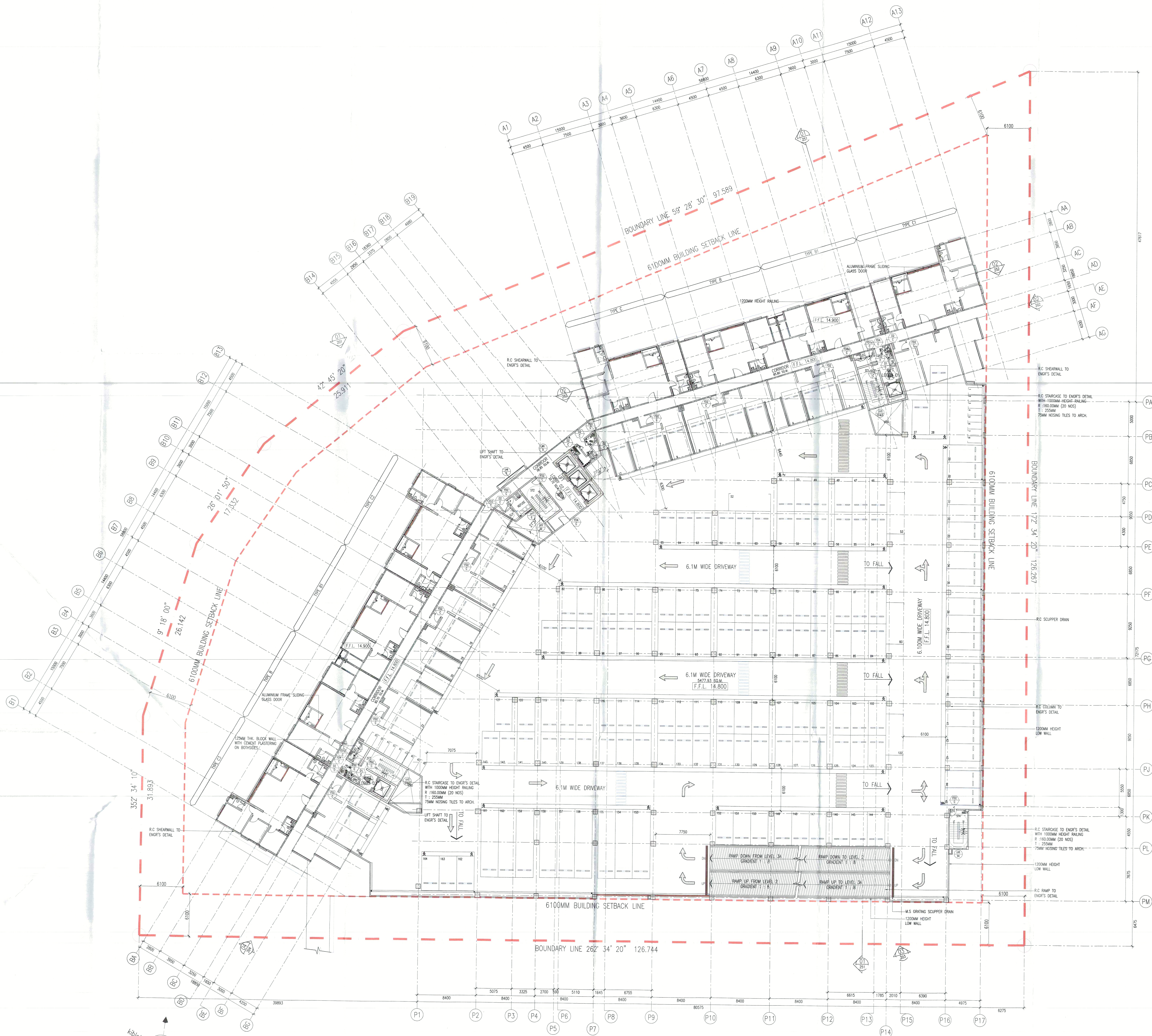
01 PELAN LANTAI ARAS 3 - 6 103 SCALE = 1 : 200
