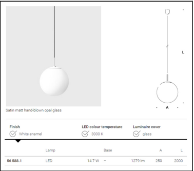
PENDANT LIGHT
