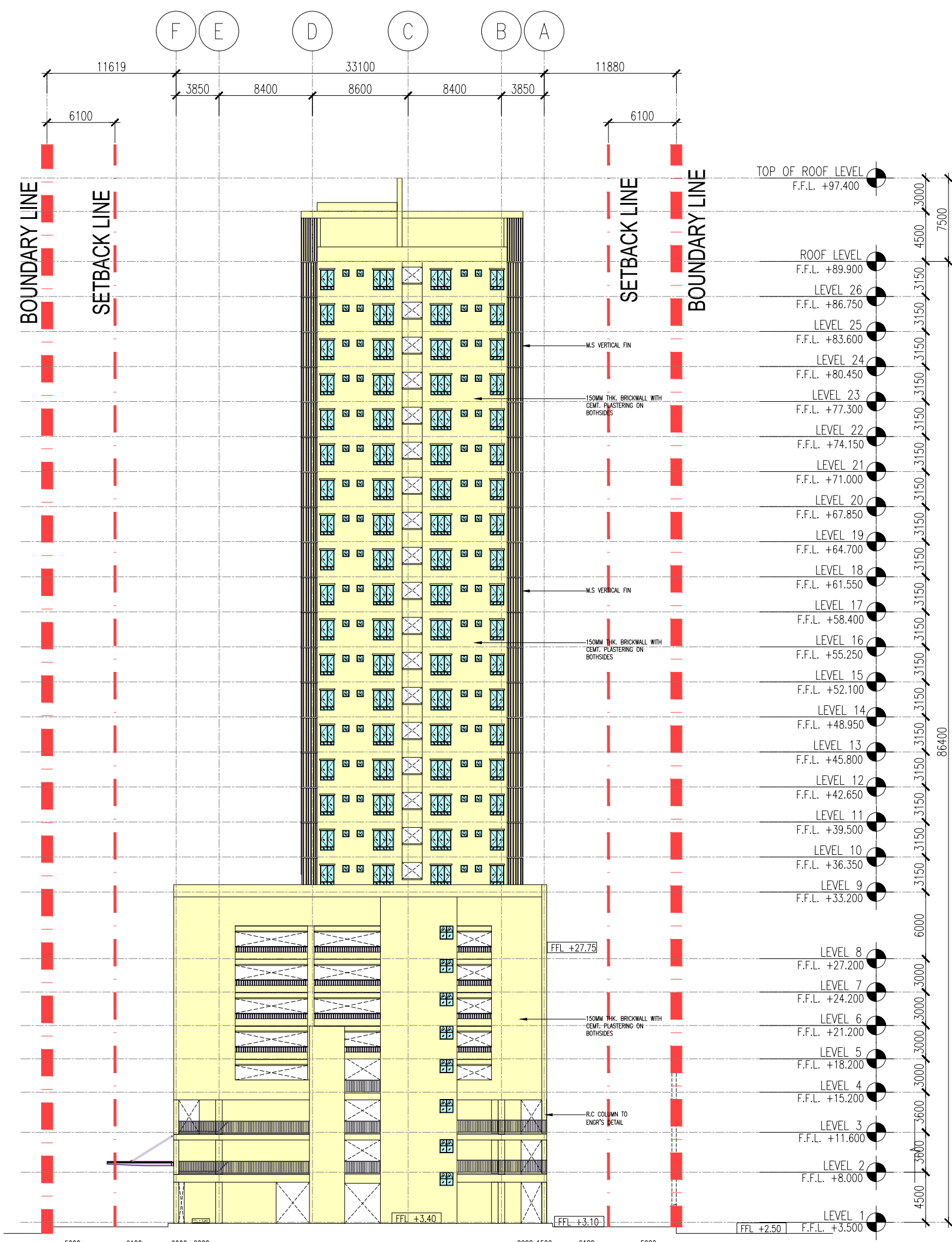
04 PANDANGAN 04 201 SKALA = 1 : 400
