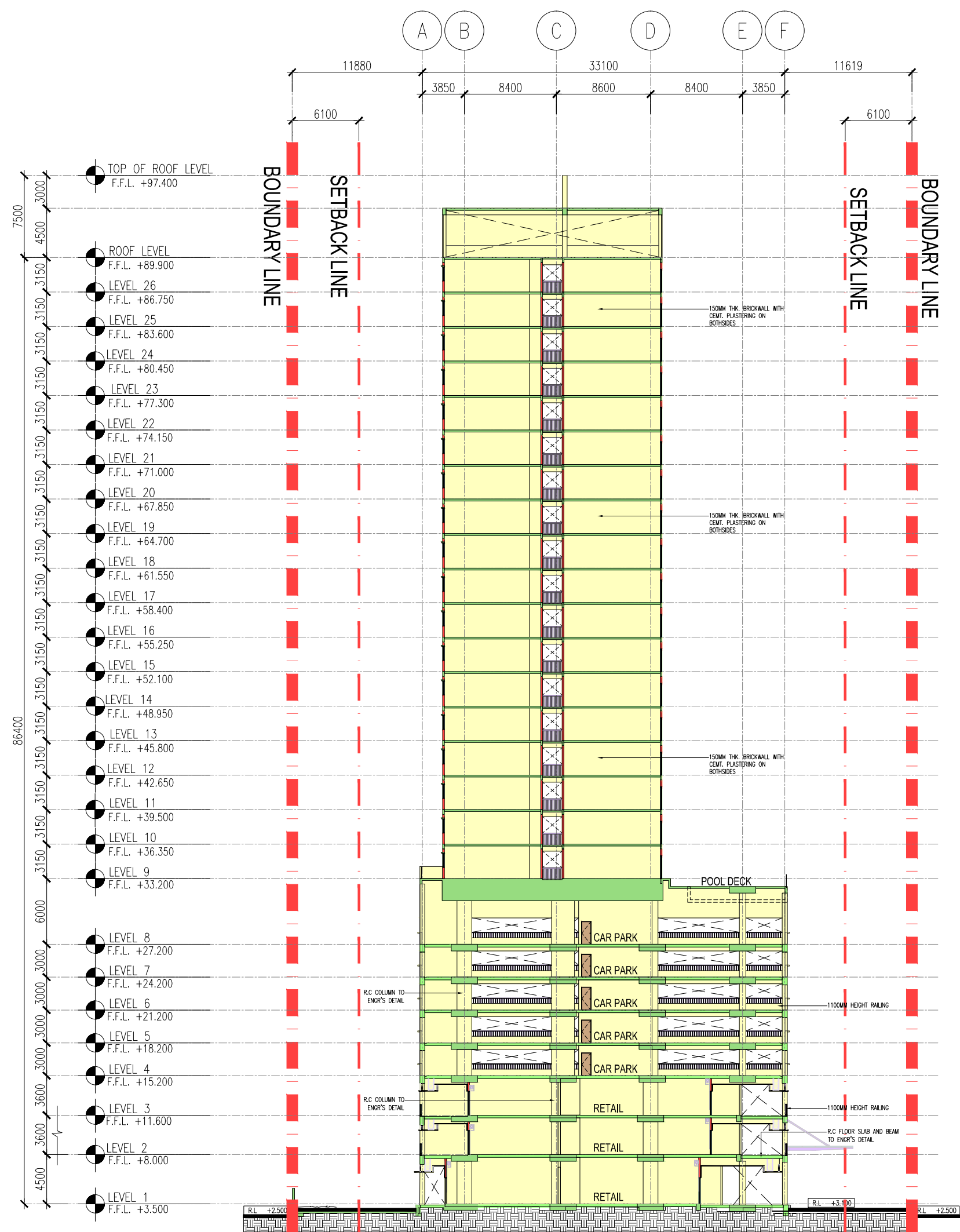
02 KERATAN 251 SKALA = 1 : 400
