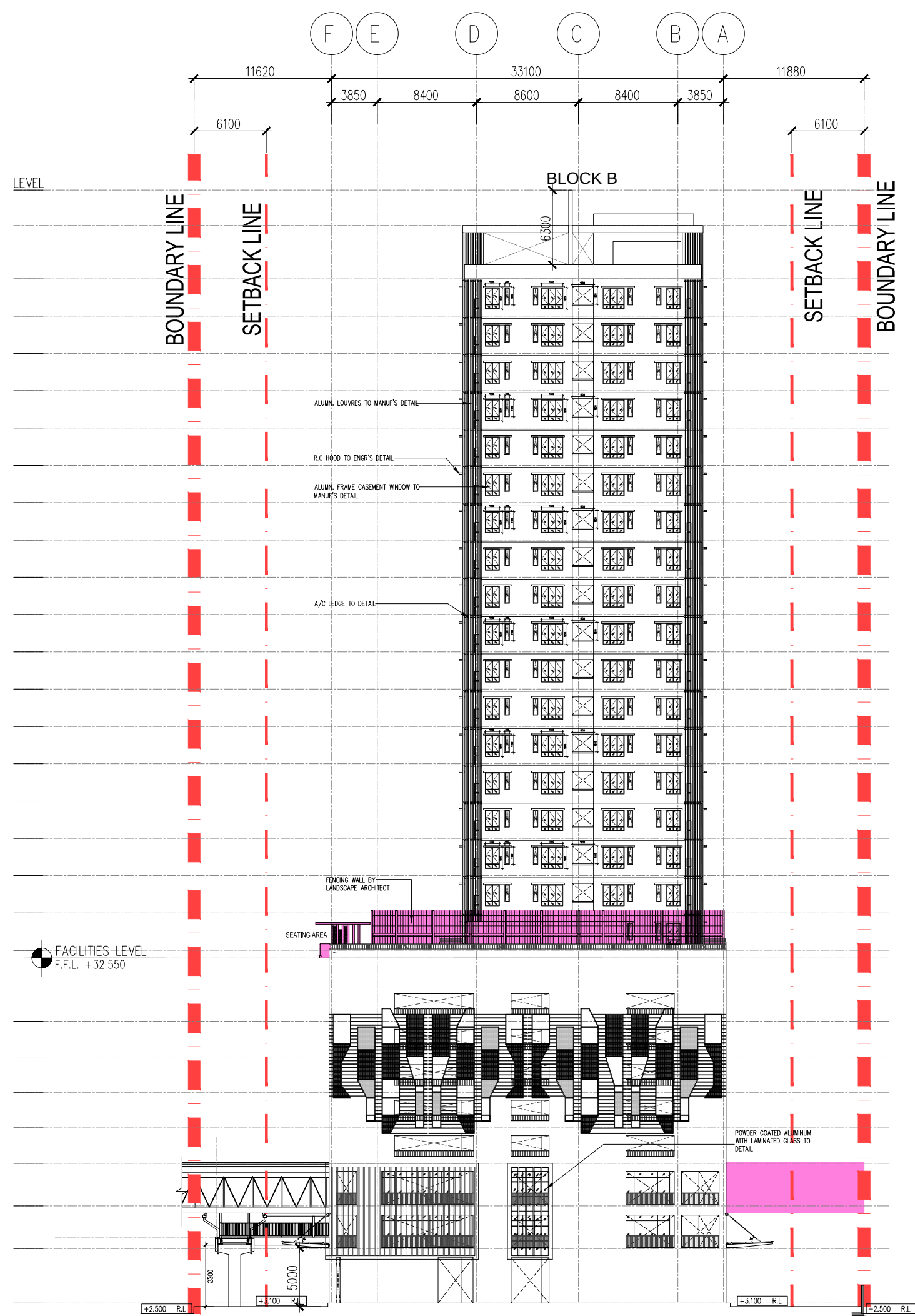
04 PANDANGAN 04 201 SKALA = 1 : 400
