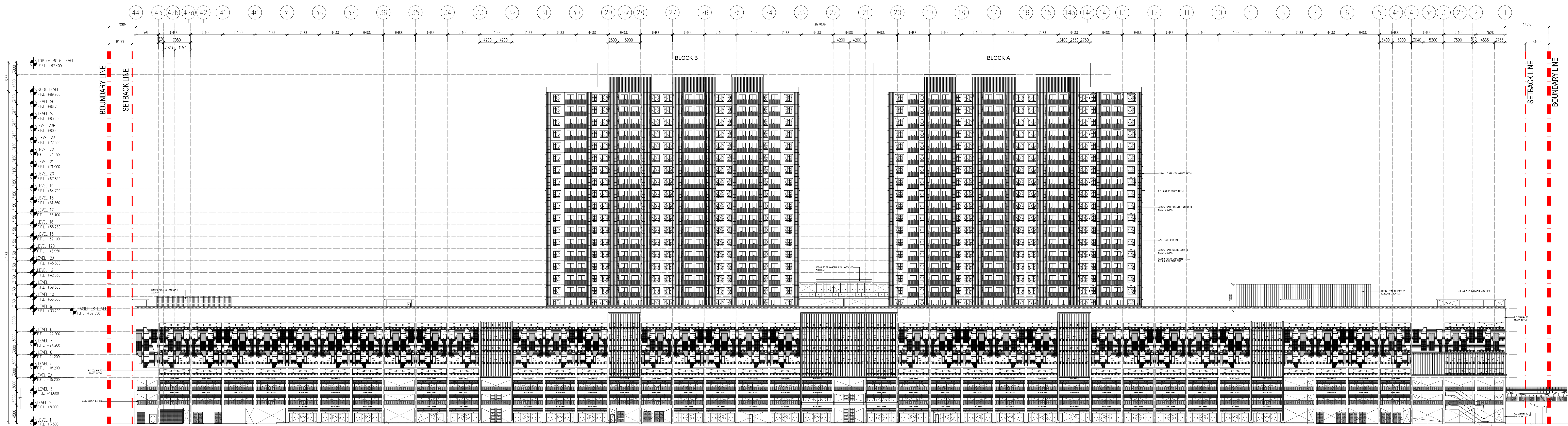
03 PANDANGAN 03 201 SKALA = 1 : 400
