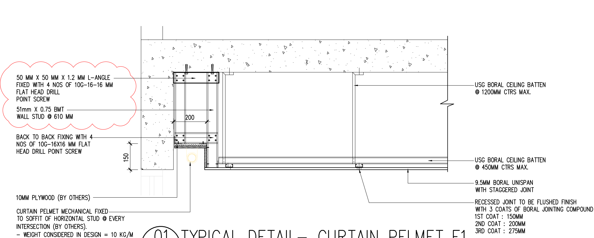
01 TYPICAL DETAIL- CURTAIN PELMET F1 710-17 SCALE = NTS
